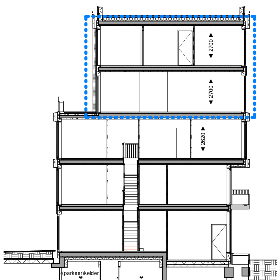
Doorsnede A-A 1 : 150
