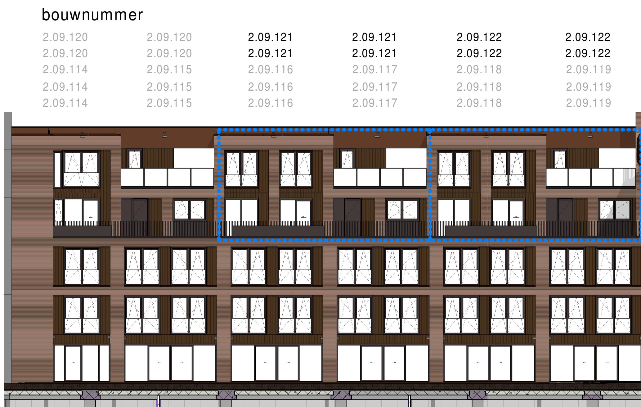
Zuid-Westgevel (Tuinzijde) 1 : 150
