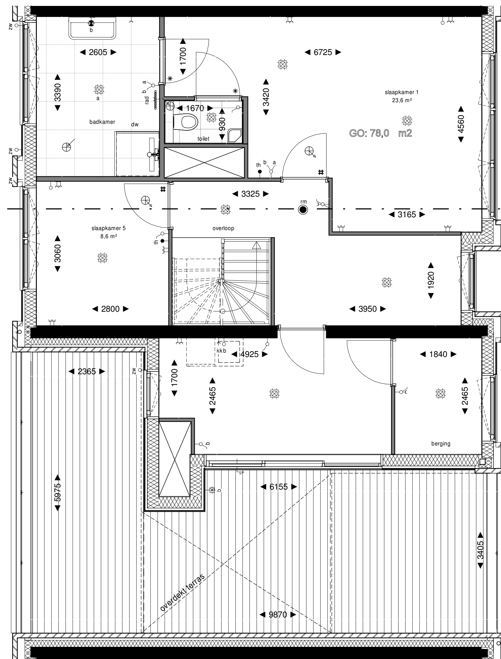
Vierde Verdieping 1 : 50
