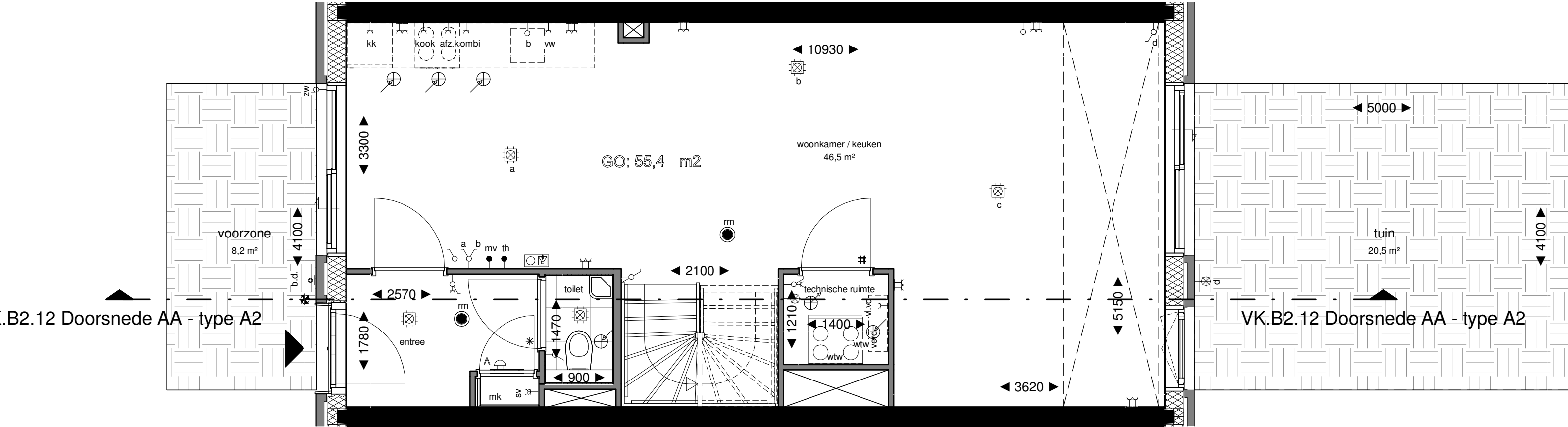
Begane Grond
