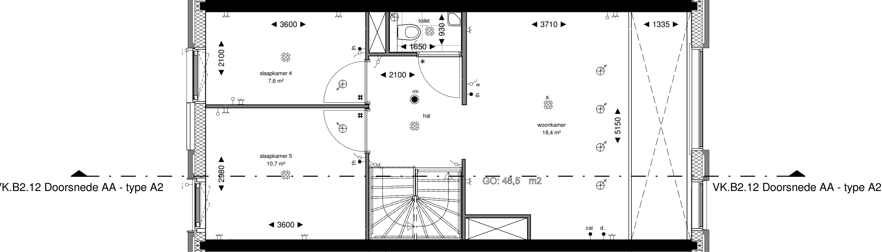
Eerste Verdieping
