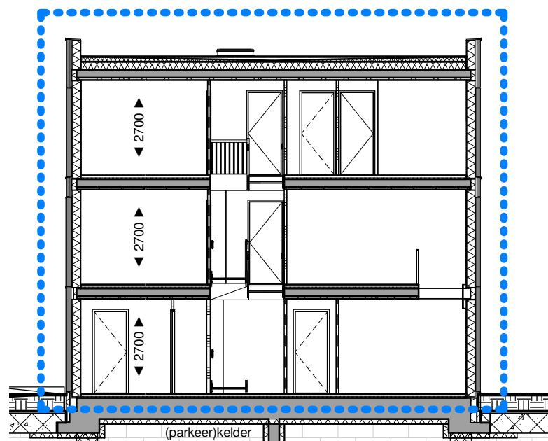
Doorsnede A-A
