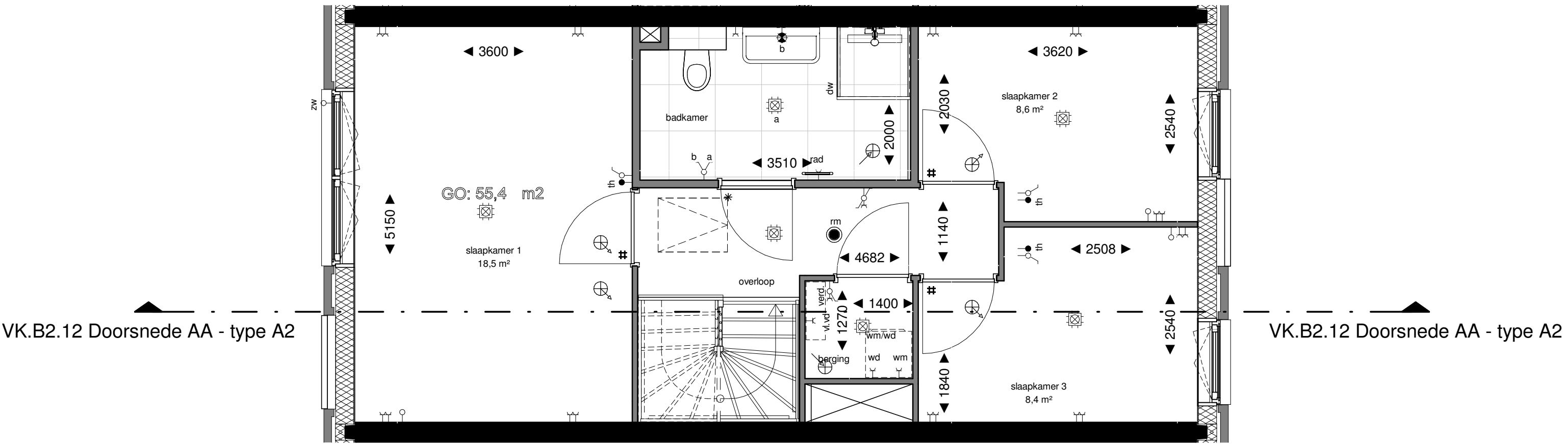
Tweede Verdieping
