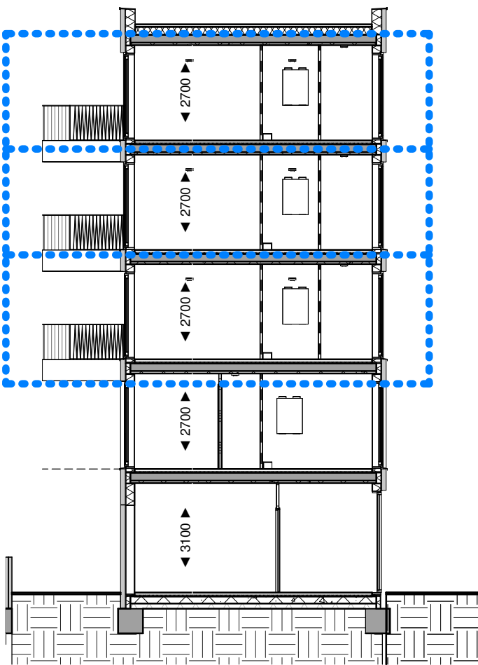
Doorsnede A-A - type C 1 : 150
