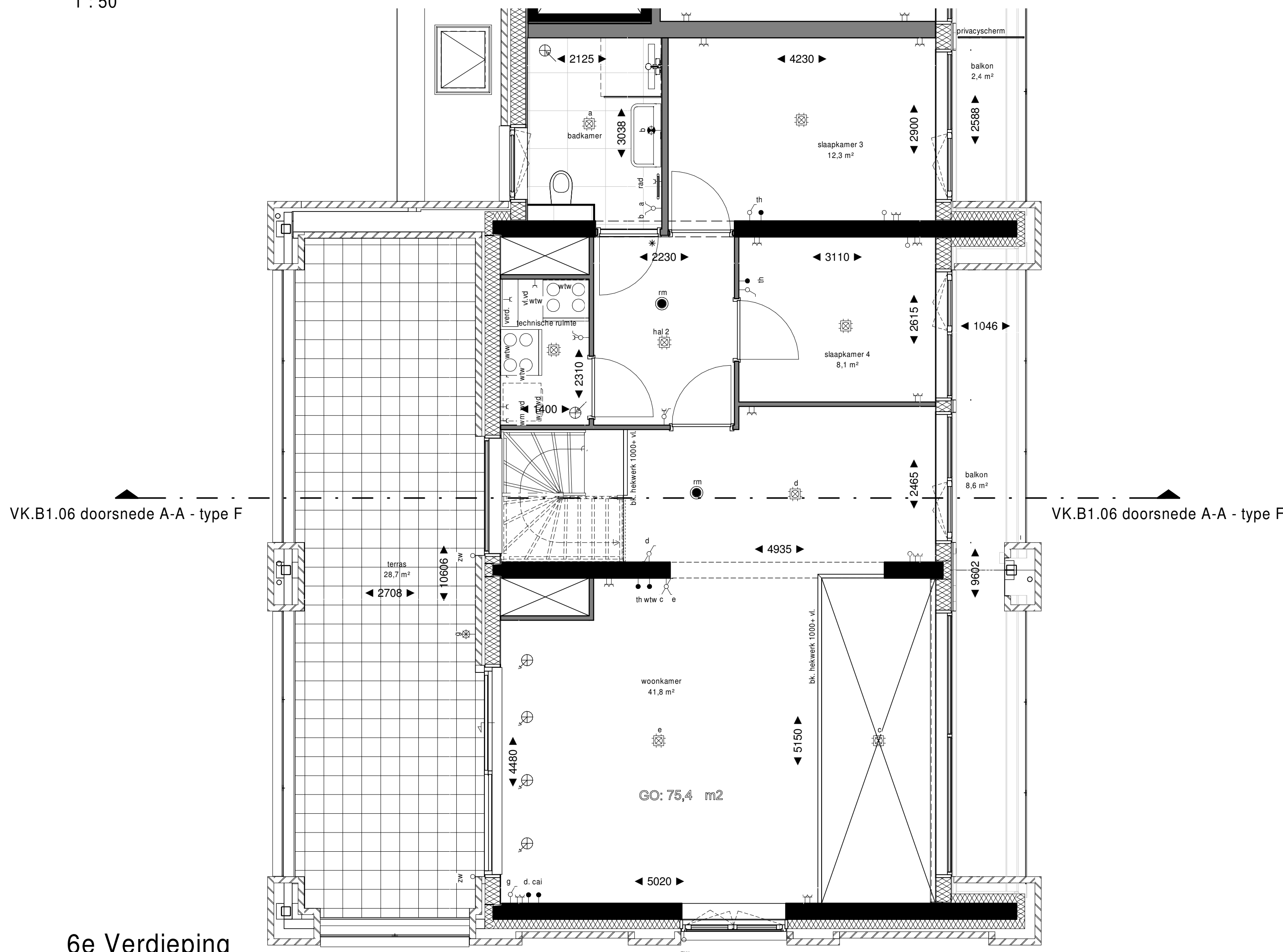
6e Verdieping
