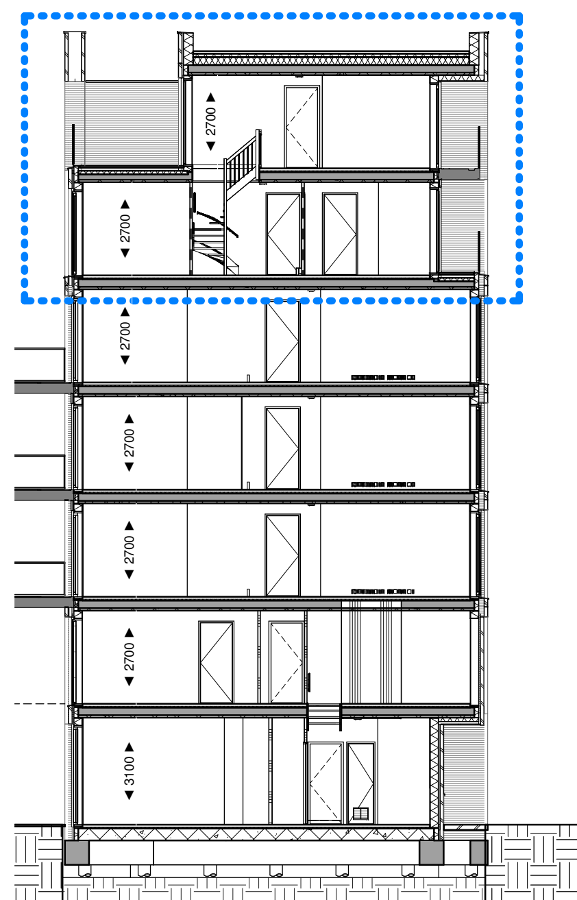
Doorsnede A-A - type F
