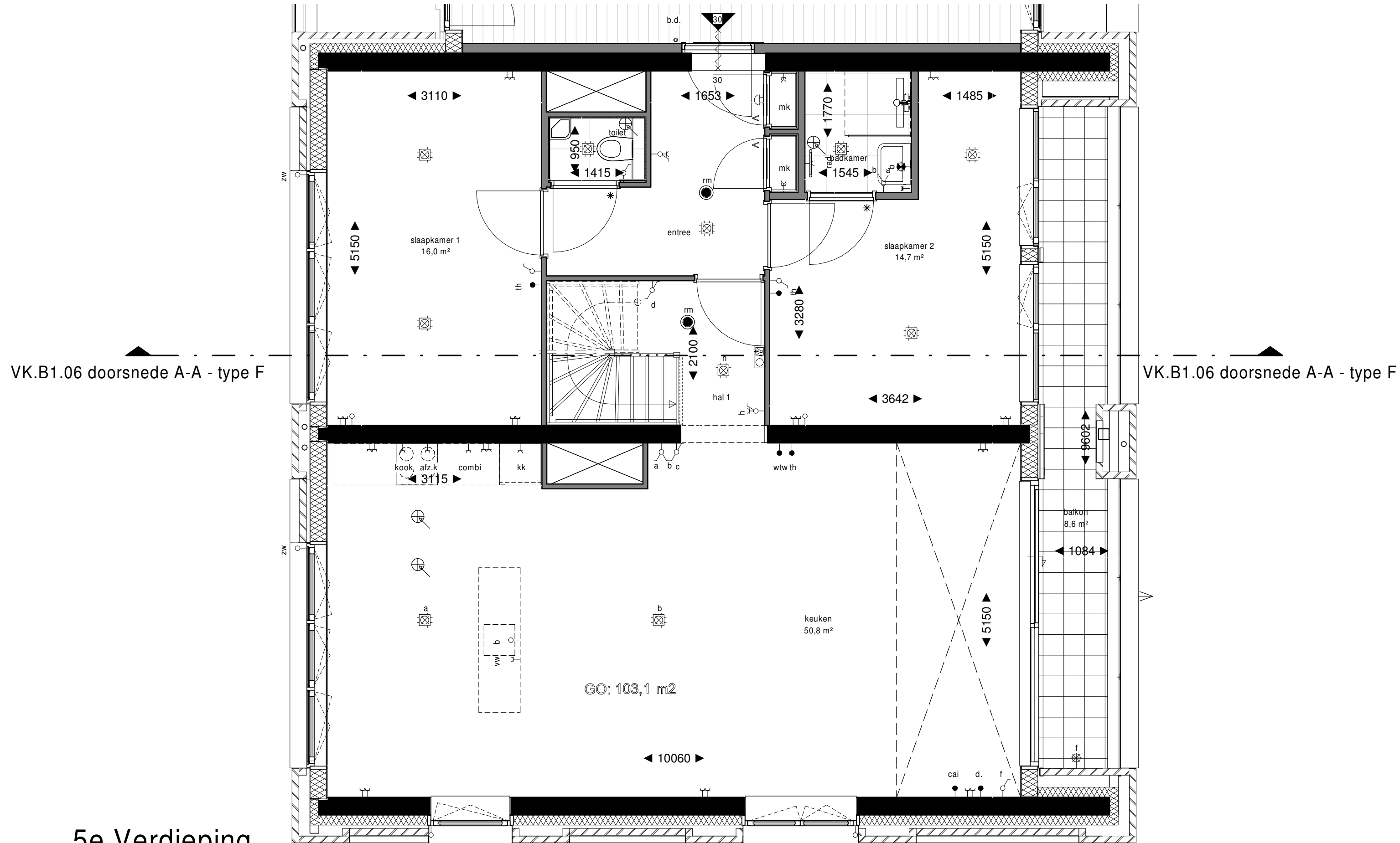
5e Verdieping
