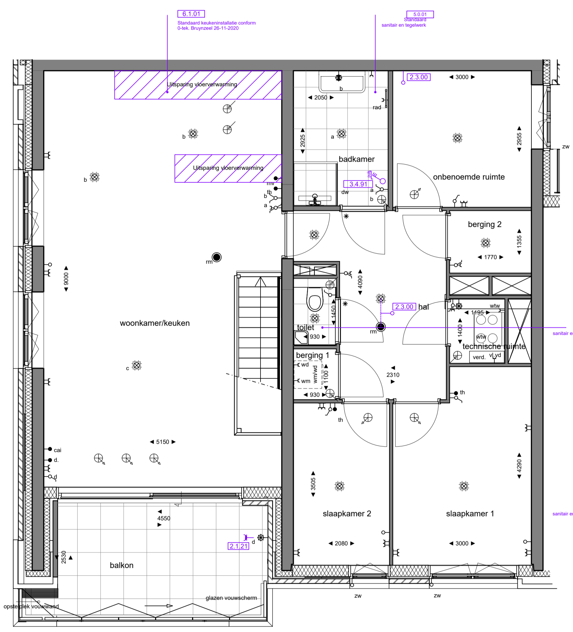
1e verdieping
