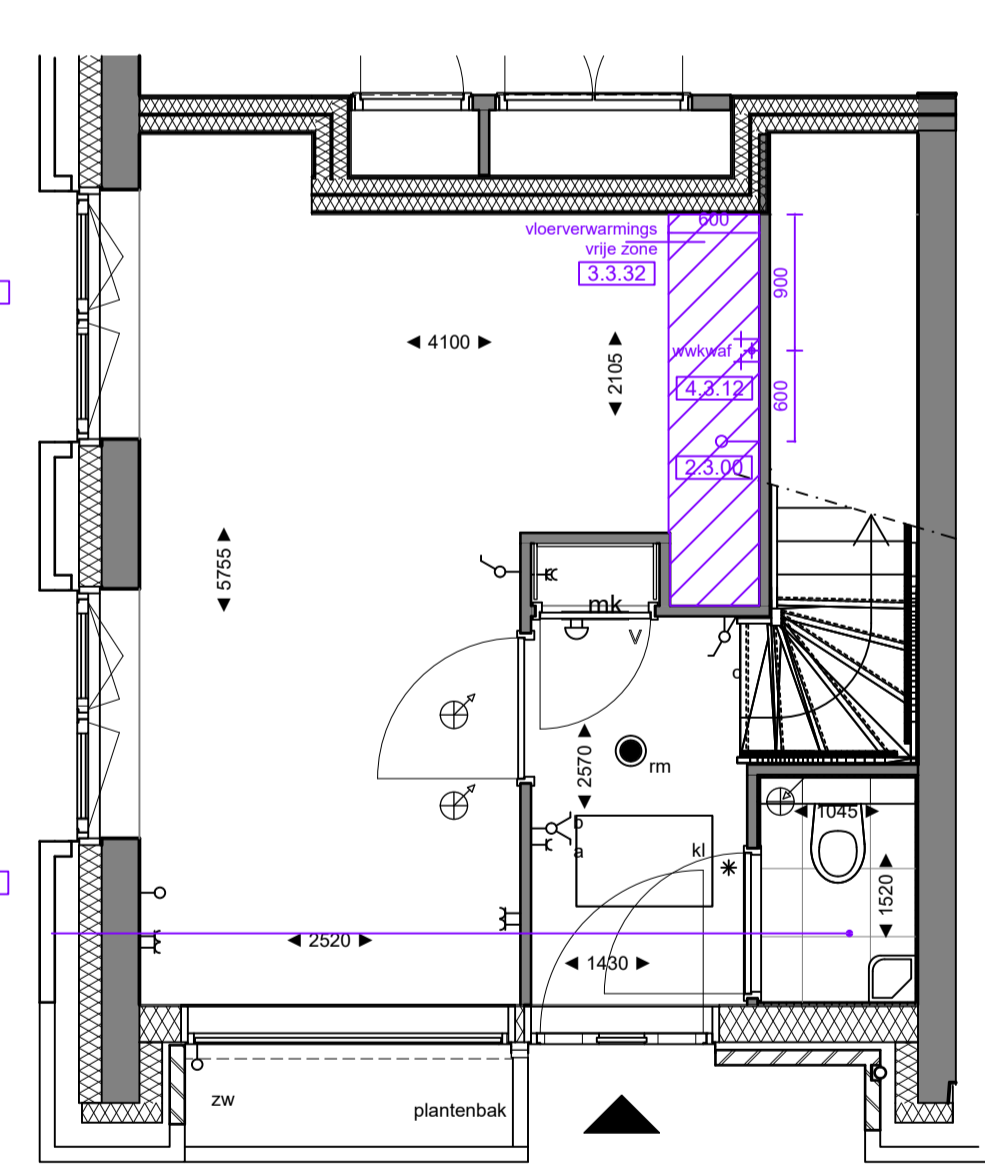
begane grond
