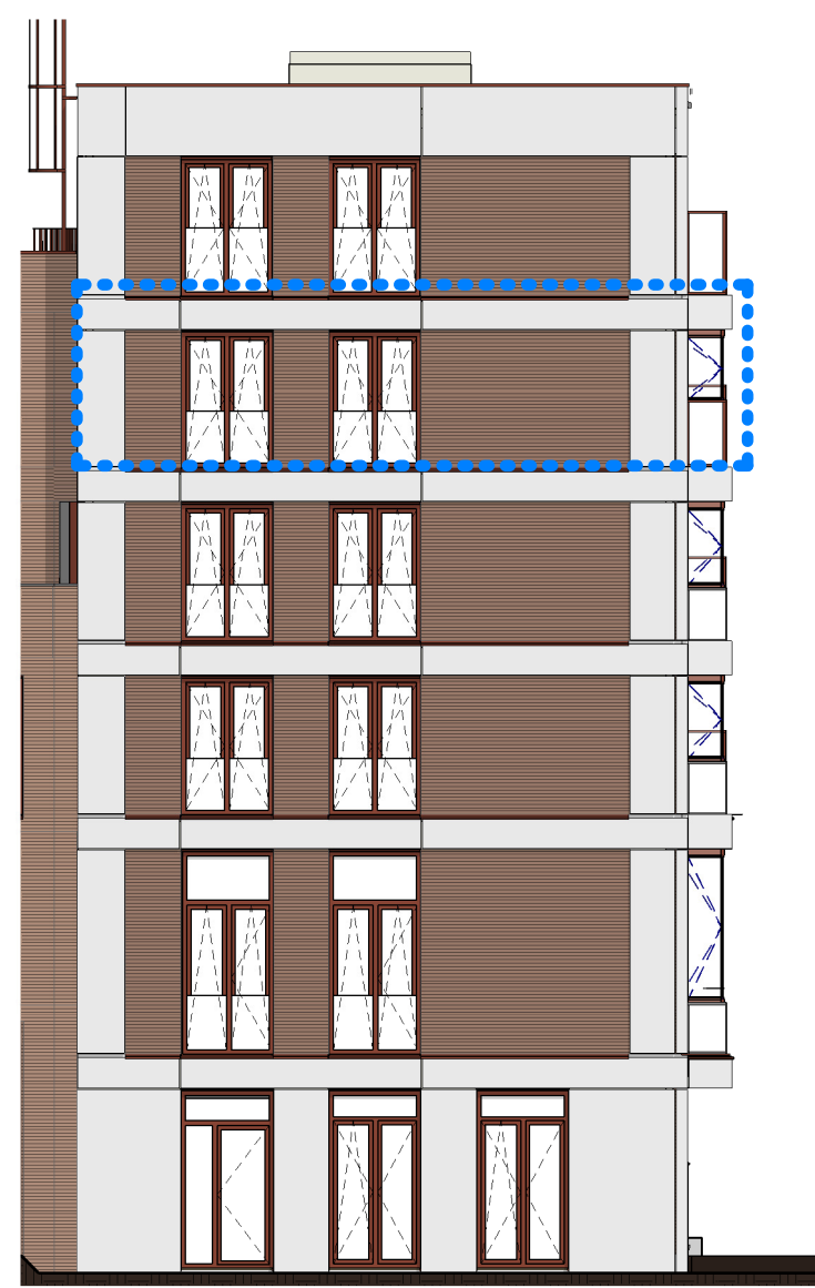
Noord-Westgevel (Zijgevel) 1 : 150
