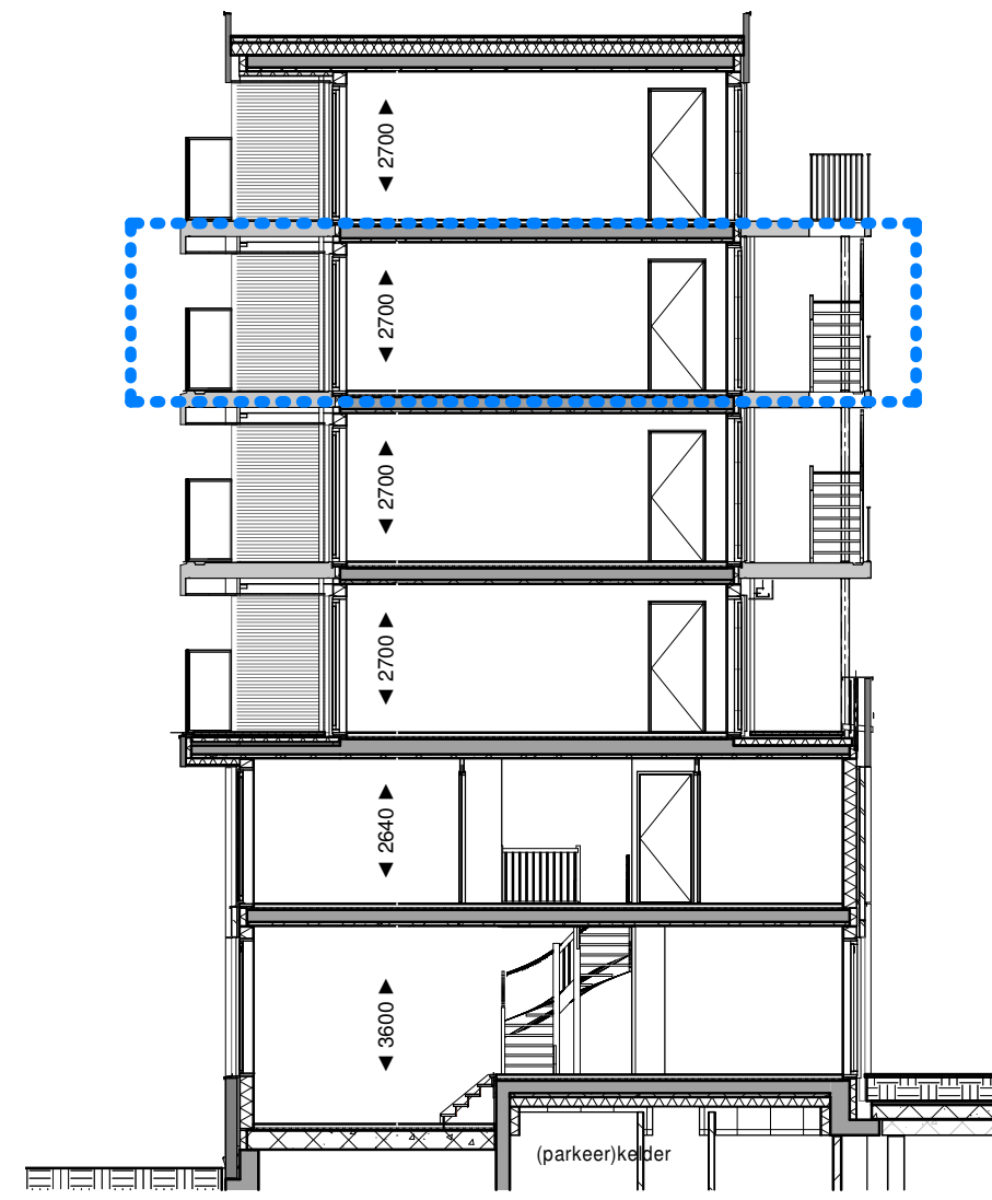
Doorsnede A-A 1 : 150
