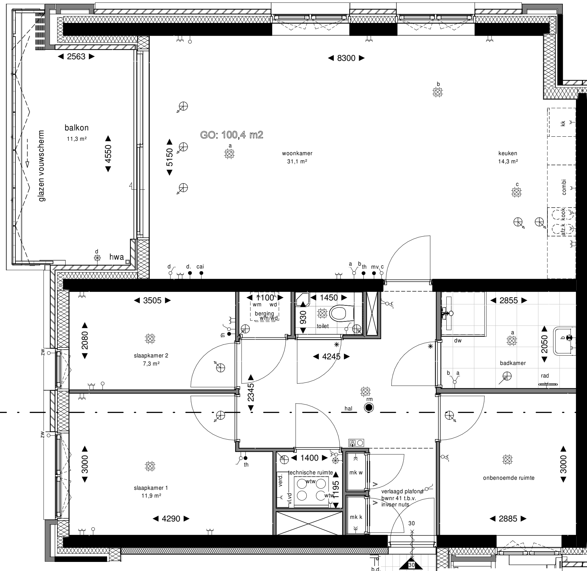
Vierde Verdieping 1 : 50
