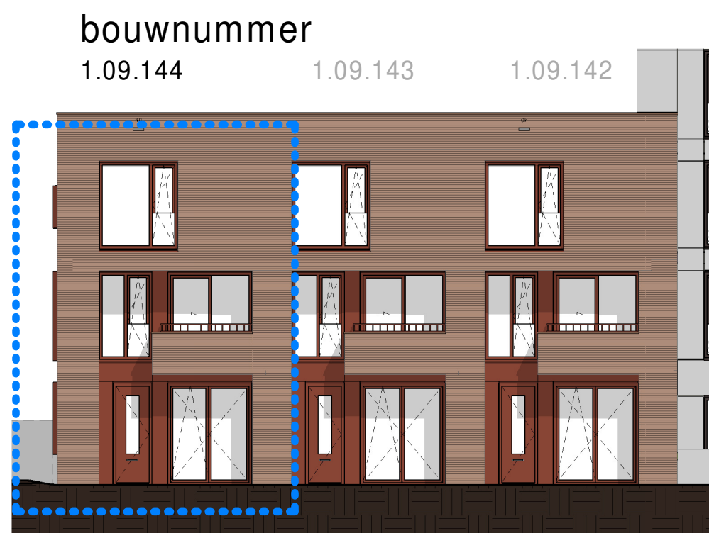
Zuid-Oostgevel (Straatzijde) 1 : 150
