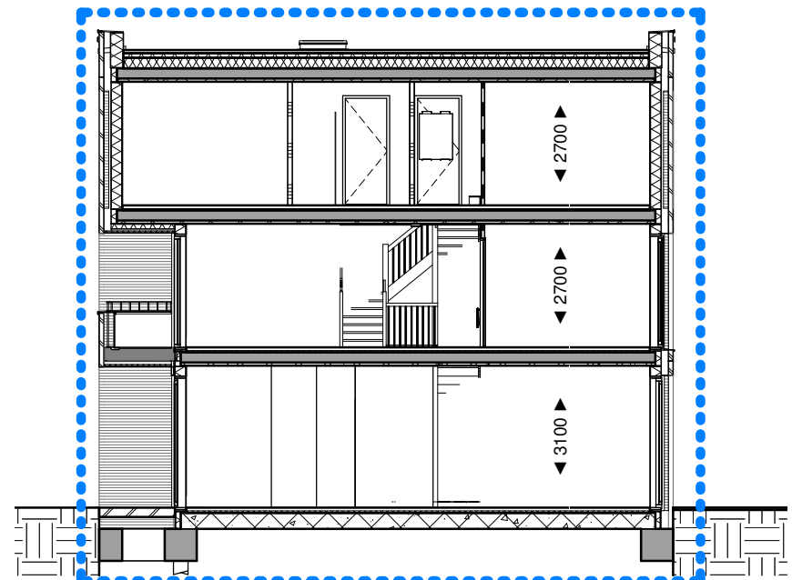
Doorsnede A-A - type A2 1 : 150
