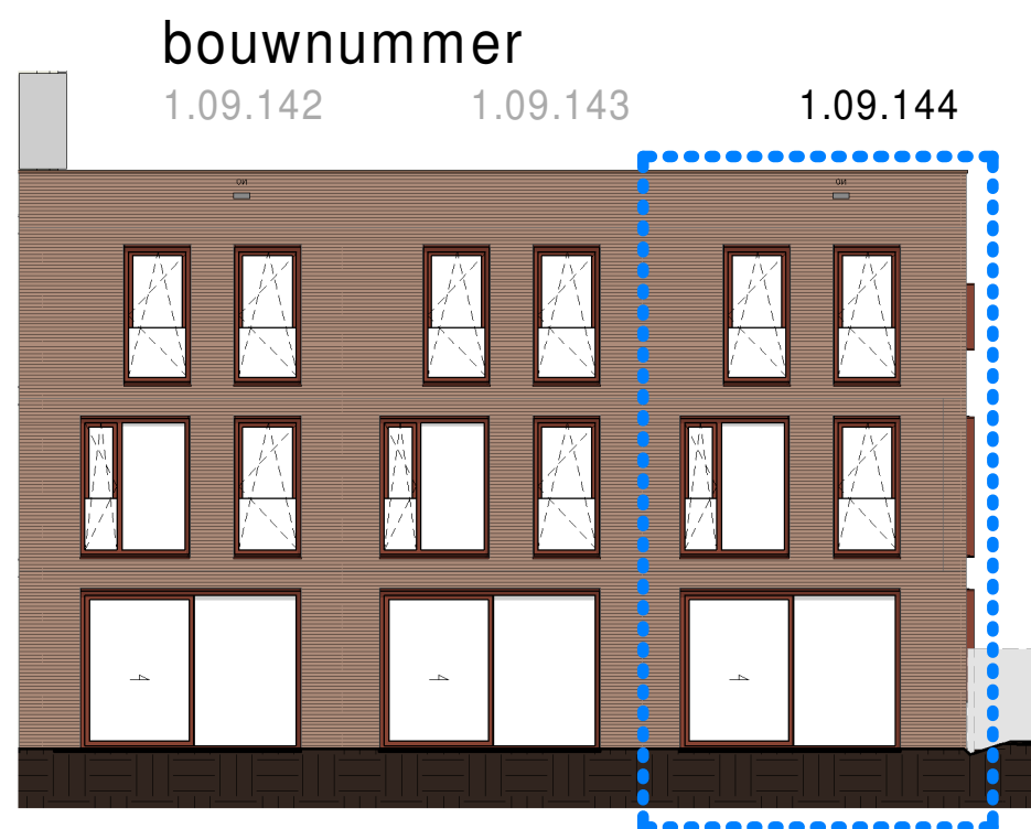
Noord-Westgevel (Tuinzijde) 1 : 150
