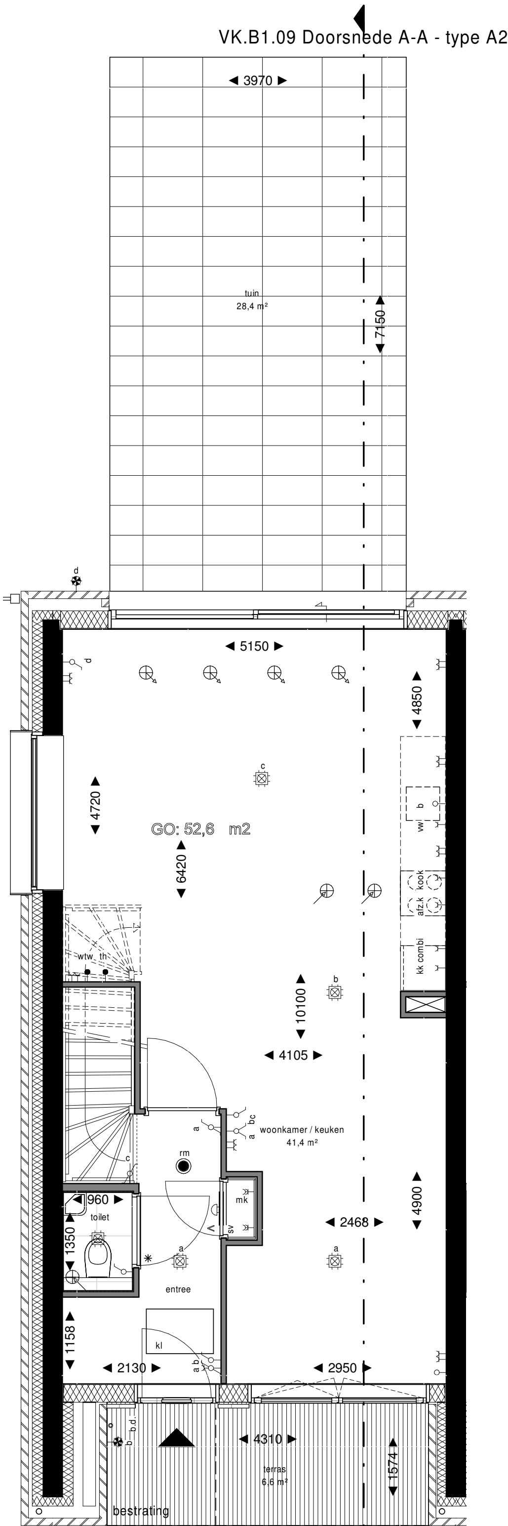
Begane Grond 1 : 50
