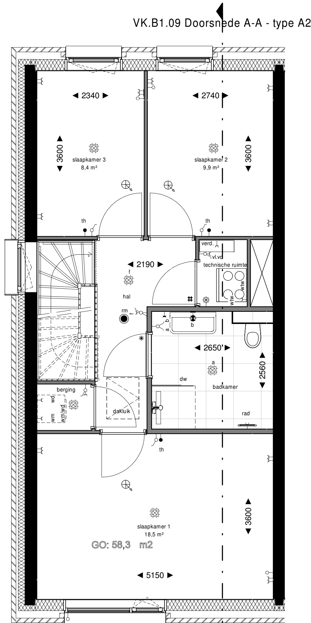
2e Verdieping 1 : 50
