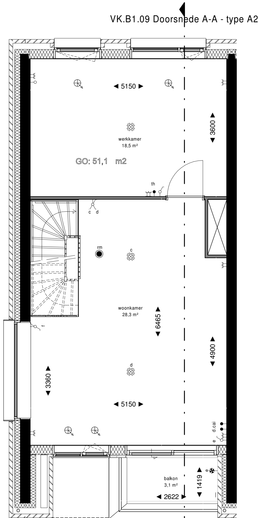
1e Verdieping 1 : 50
