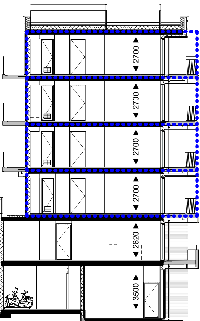
Doorsnede A-A
