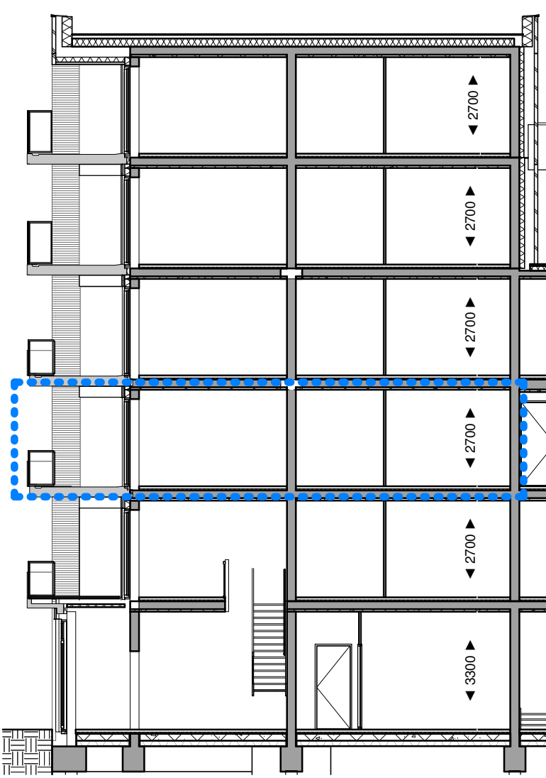
Doorsnede A-A 1 : 150
