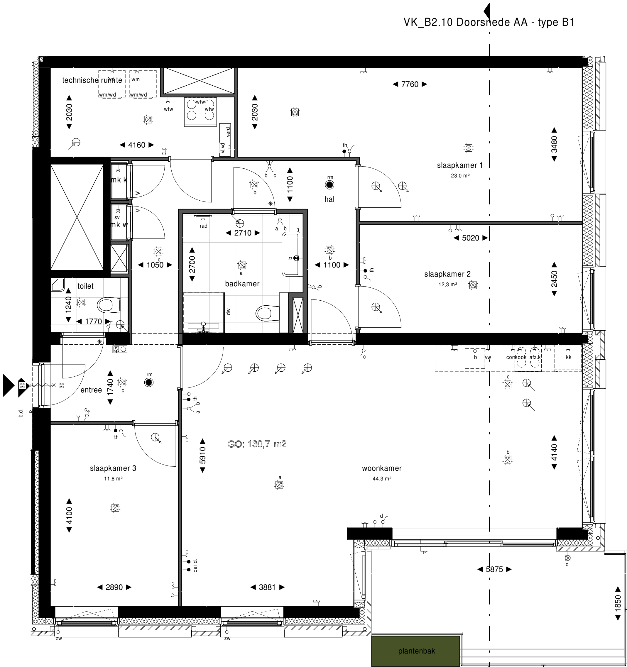
Tweede Verdieping 1 : 50
