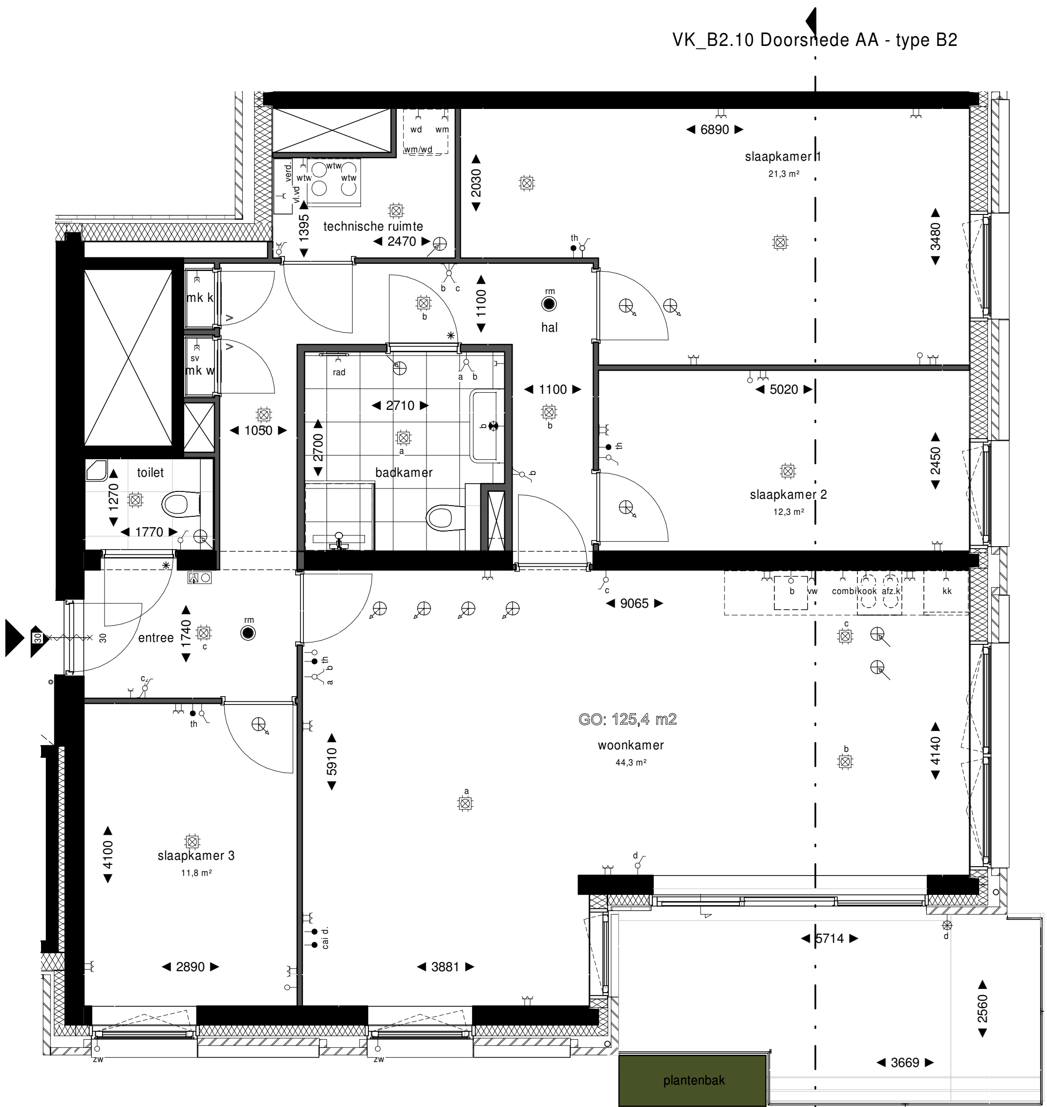
Derde Verdieping 1 : 50
