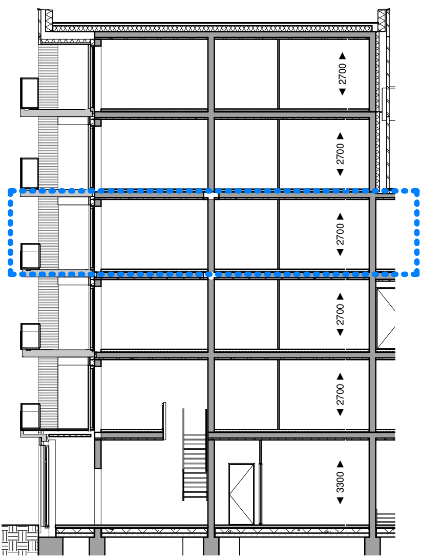
Doorsnede A-A 1 : 150
