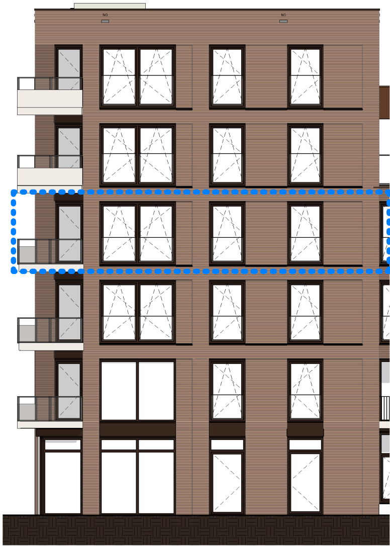
Noord-Oostgevel (Straatzijde) 1 : 150
