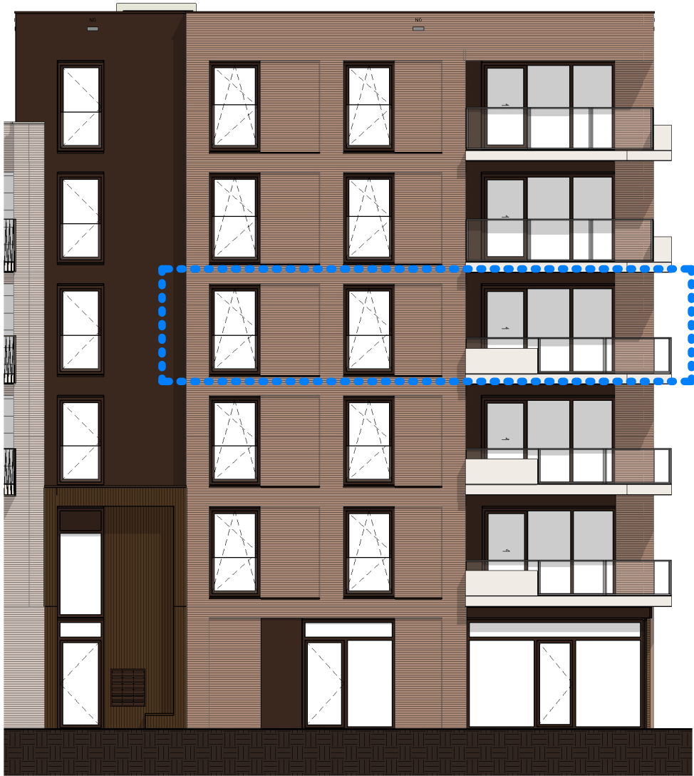
Zuid-Oostgevel (Straatzijde) 1 : 150
