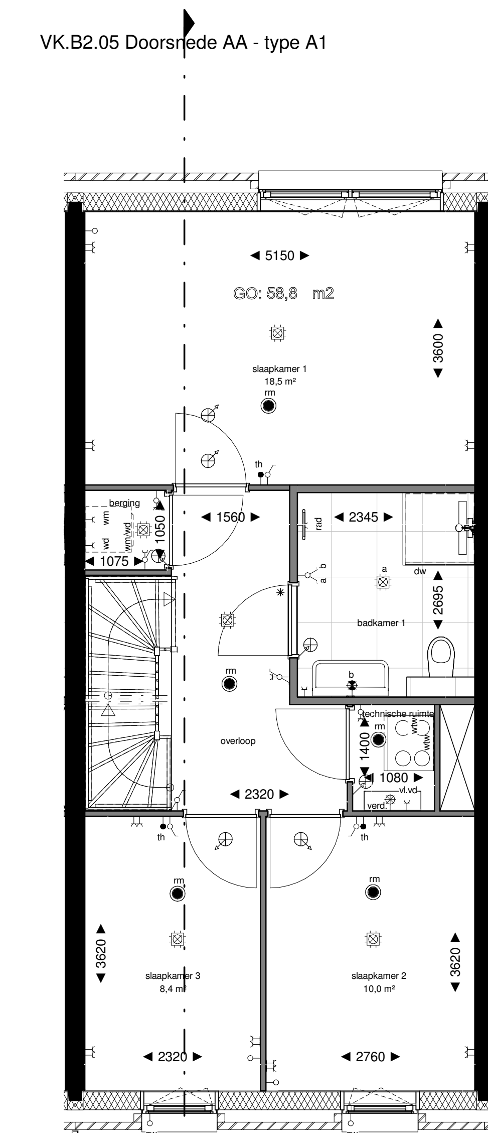
Tweede Verdieping 1 : 50
