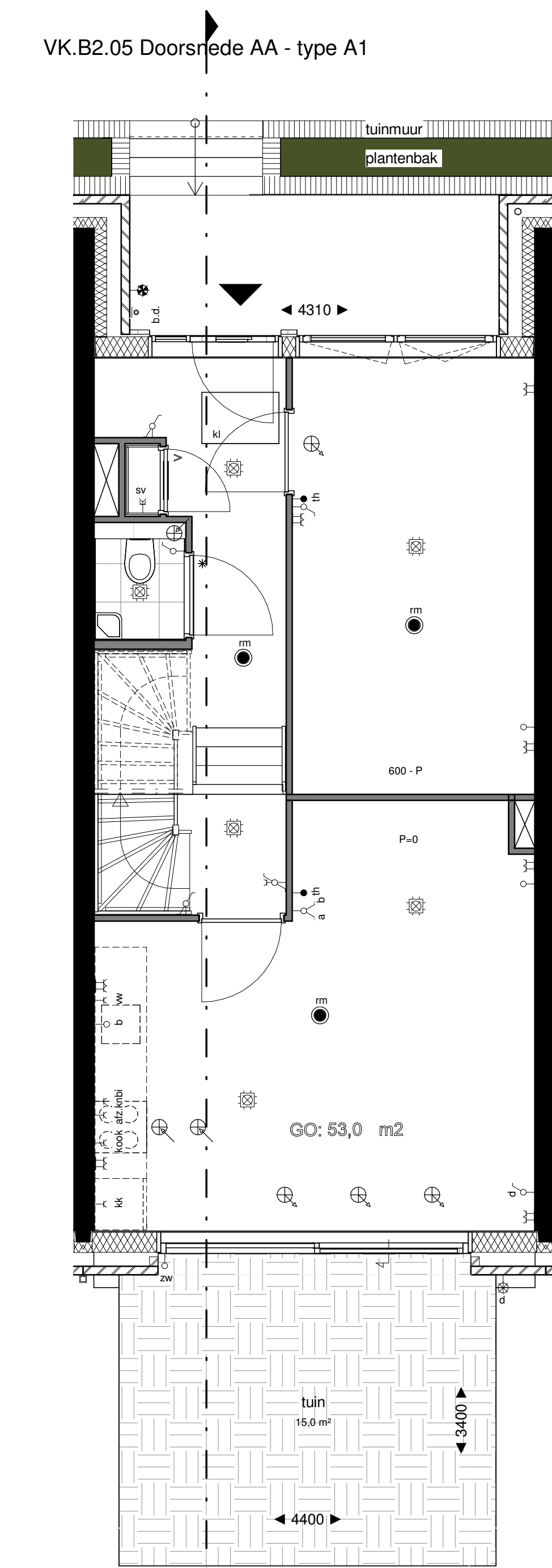
Begane Grond 1 : 50
