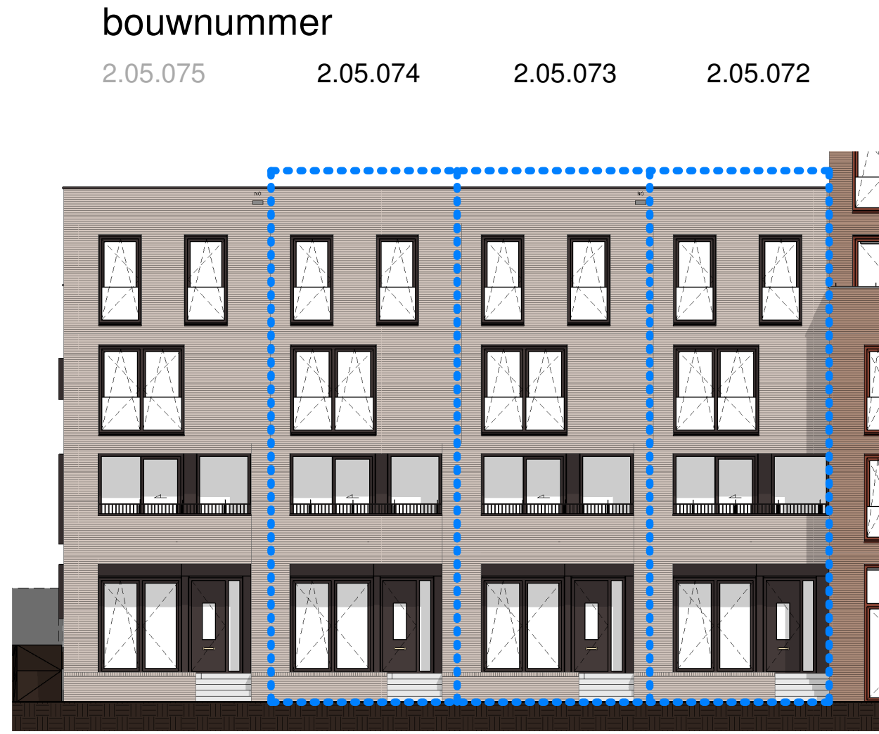
Noord-Westgevel (Straatzijde) 1 : 150
