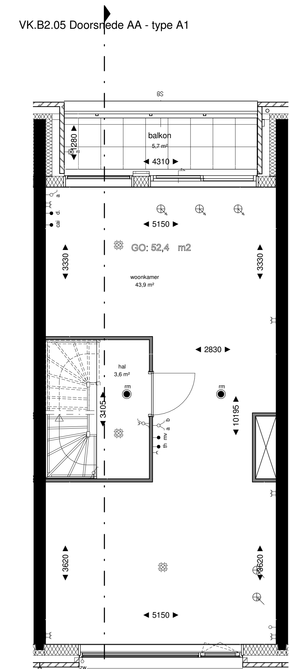
Eerste Verdieping 1 : 50
