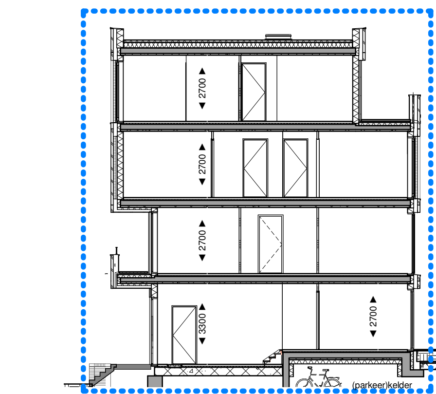
Doorsnede A-A 1 : 150
