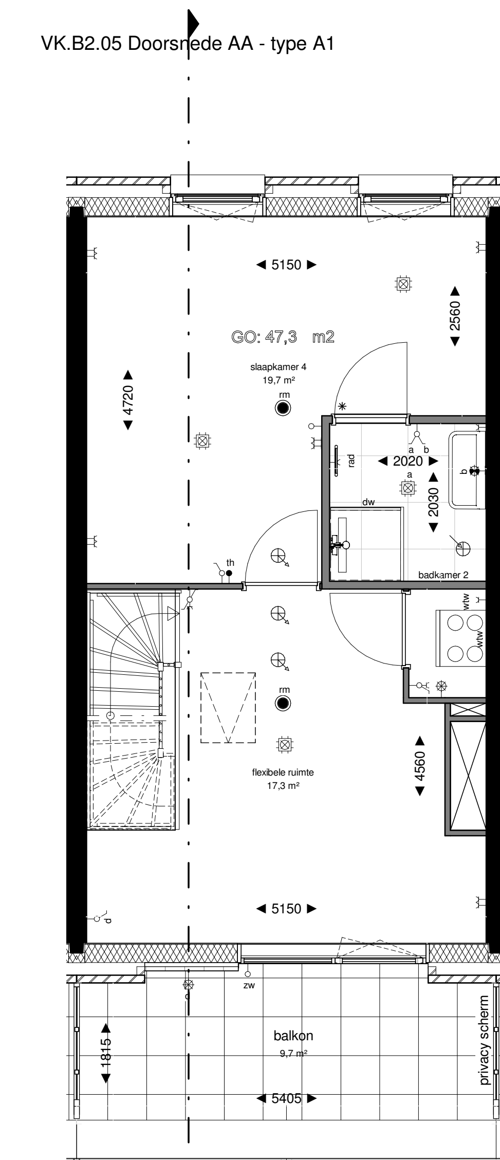
Derde Verdieping 1 : 50
