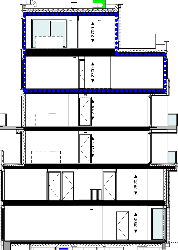
Doorsnede A-A
