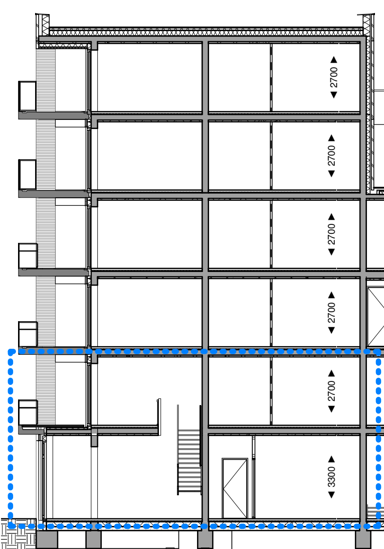
Doorsnede A-A
