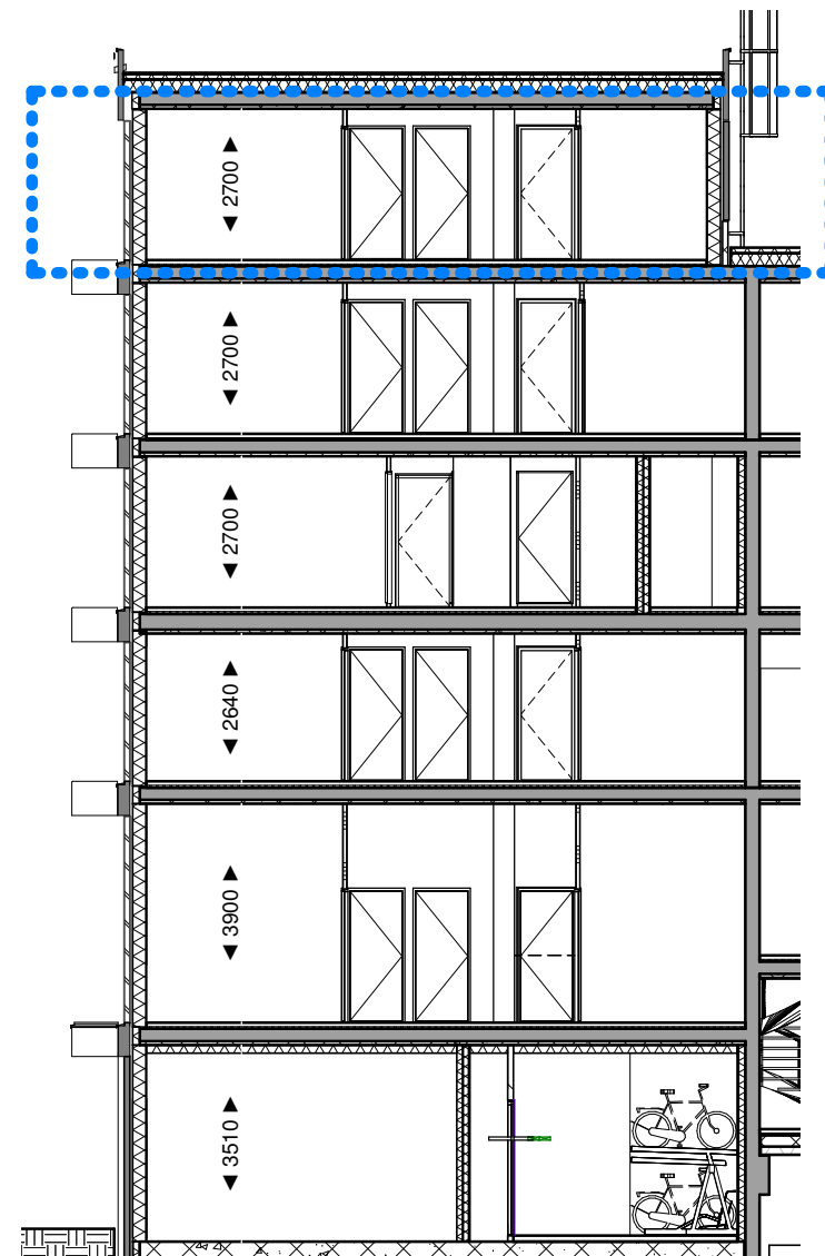
Doorsnede A-A
