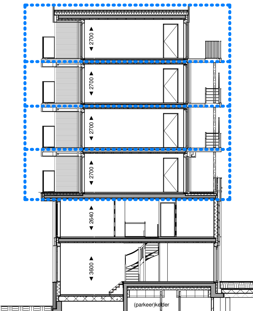
Doorsnede A-A
