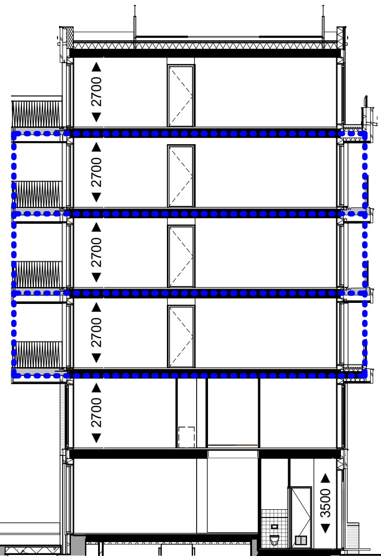
Doorsnede A-A
