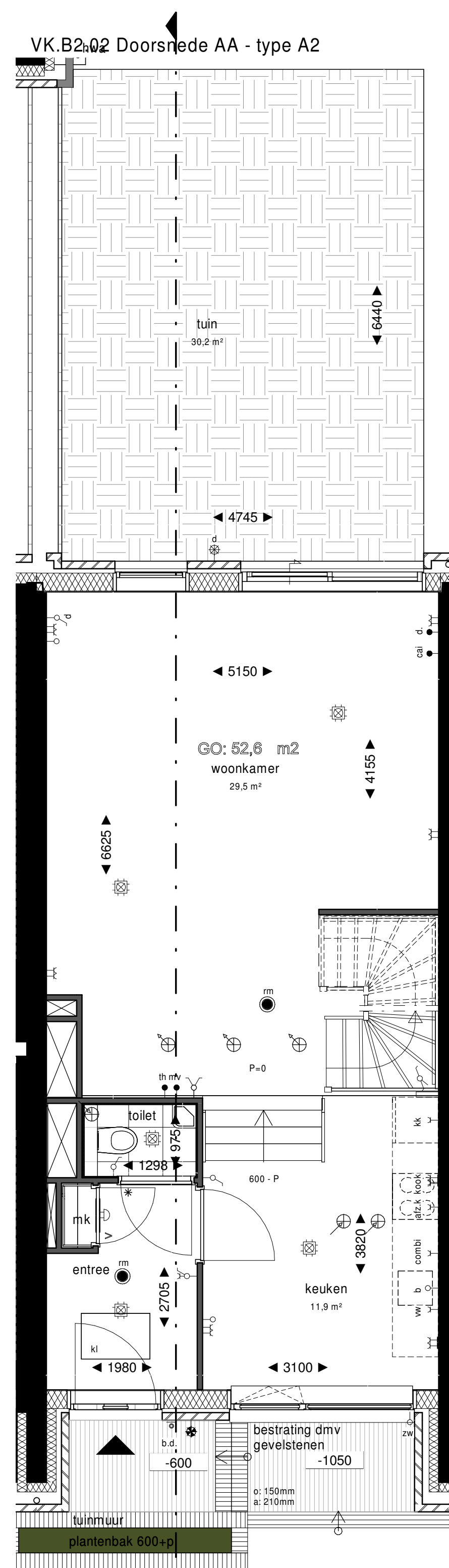
VK.B2.02 Doorsnede AA - type A2
