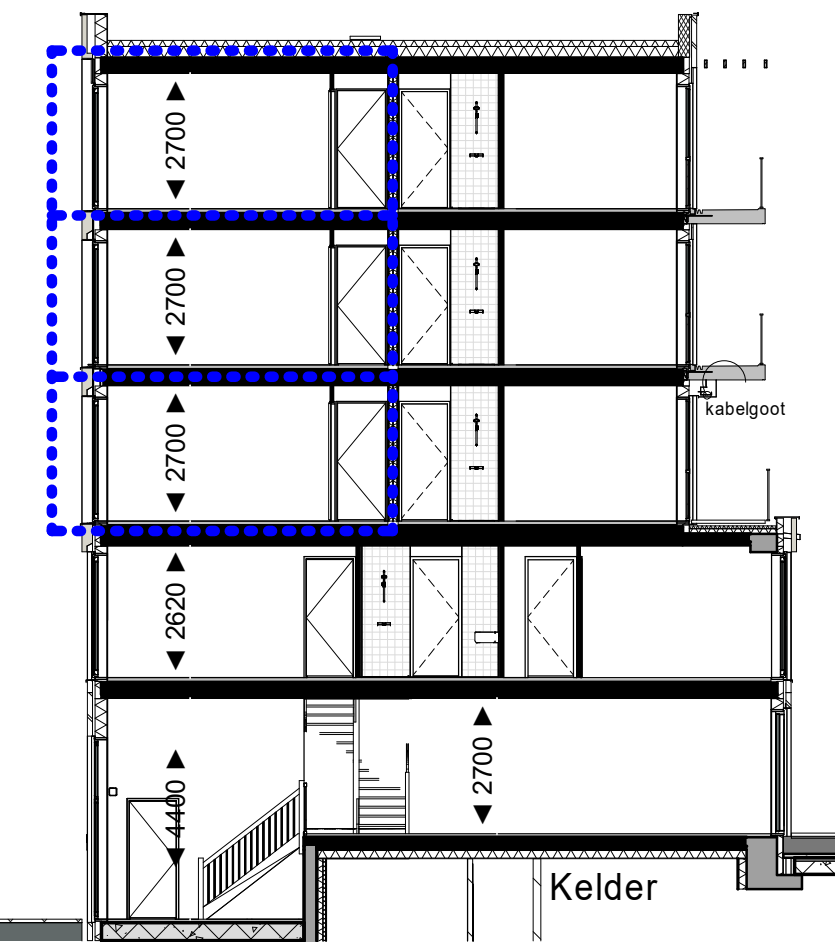
Doorsnede A-A
