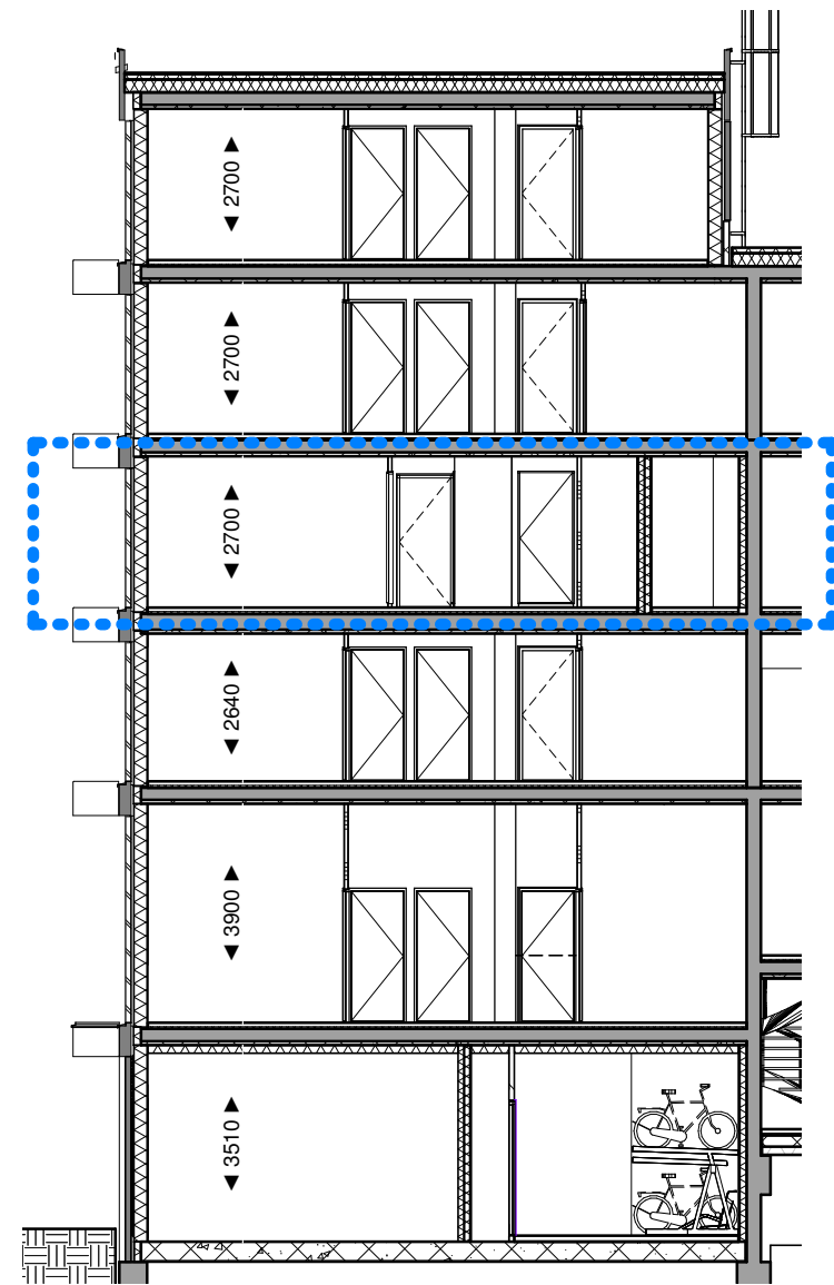
Doorsnede A-A
