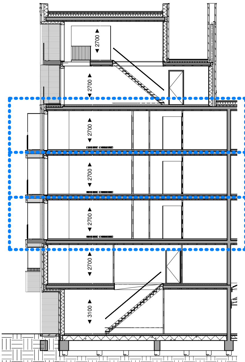
Doorsnede A-A - type C
