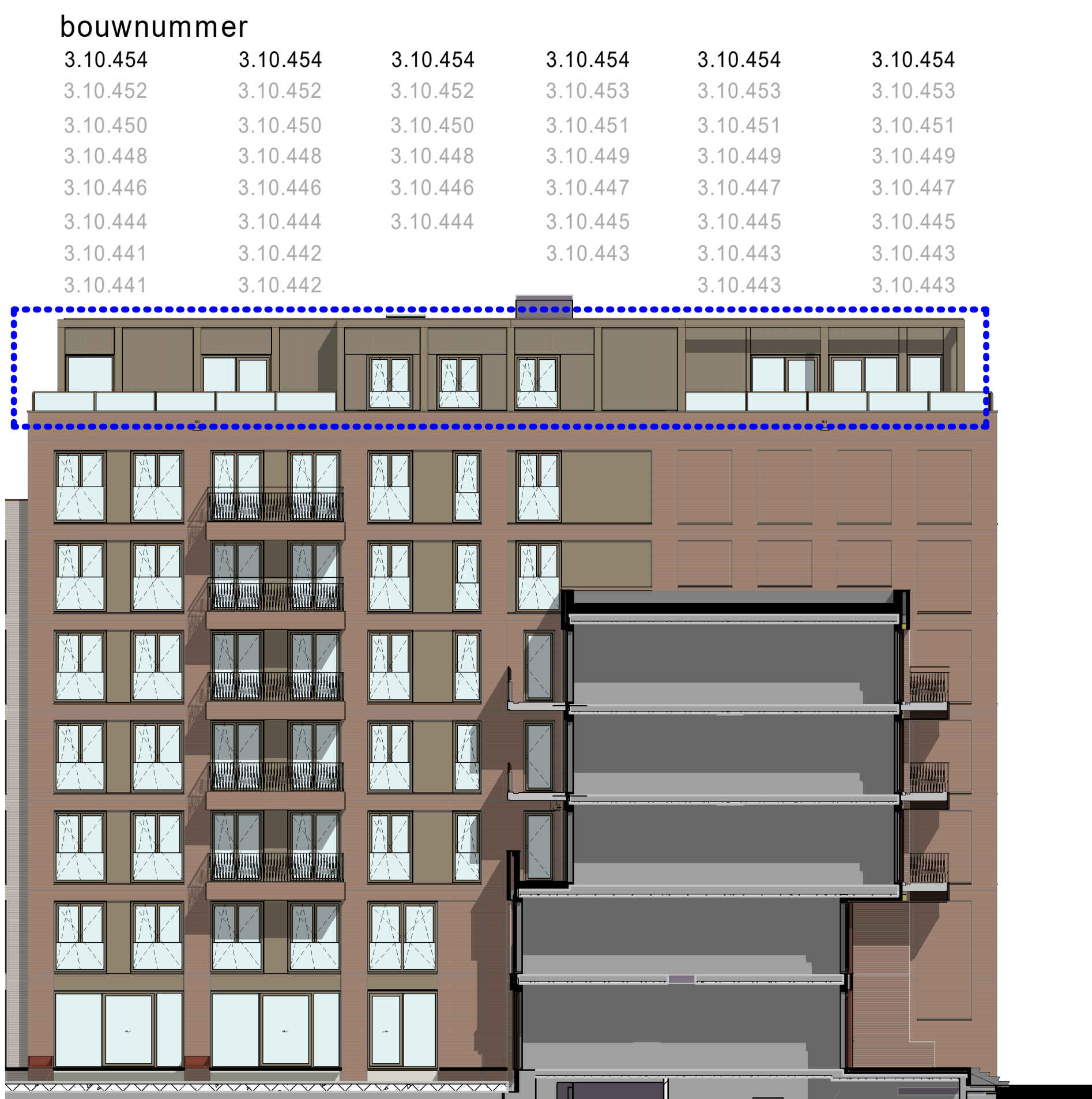
Zuid-Westgevel (Tuintzijde) 1 : 150
