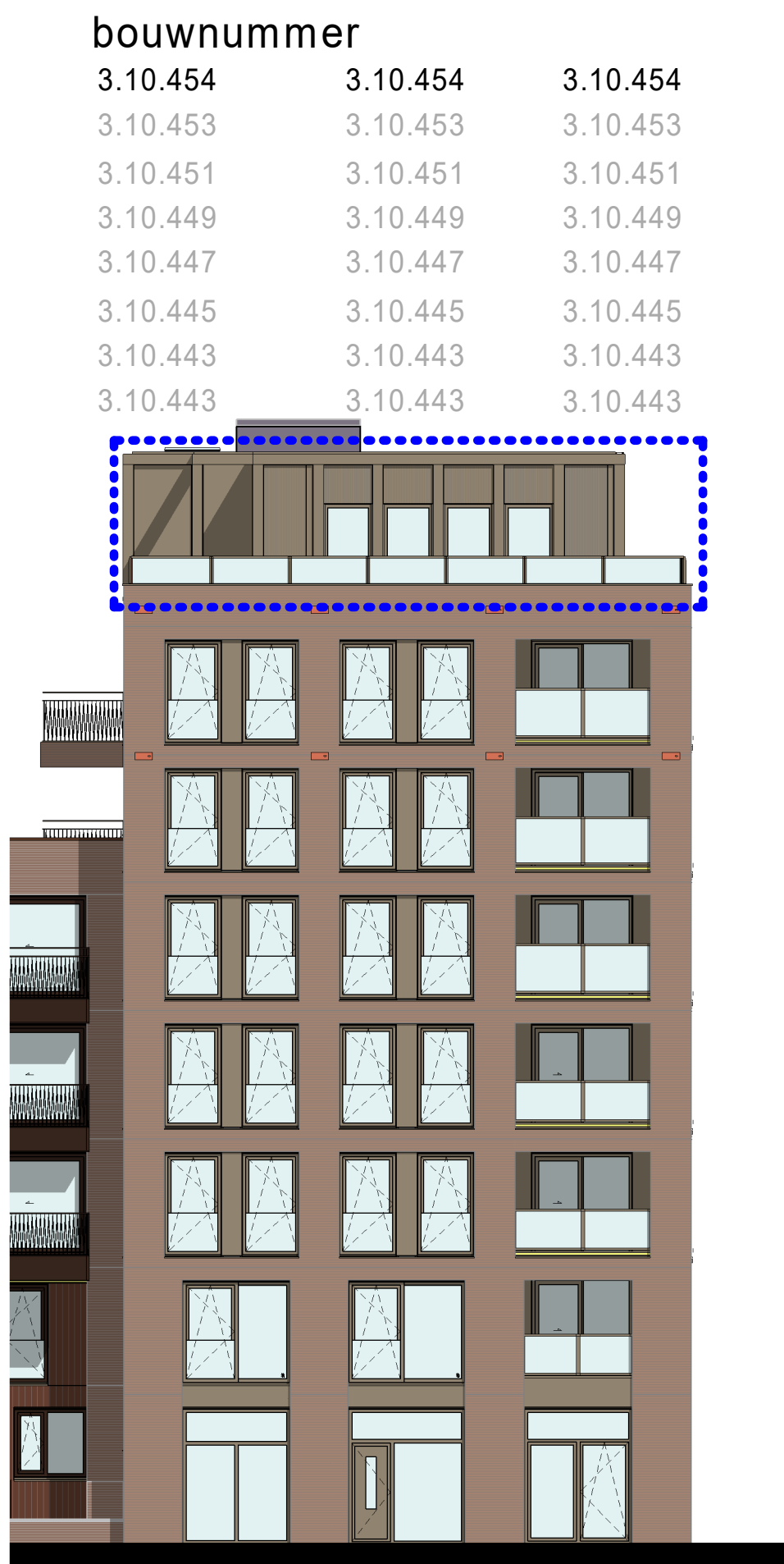
Zuid-Oostgevel (Stratzijde) 1 : 150
