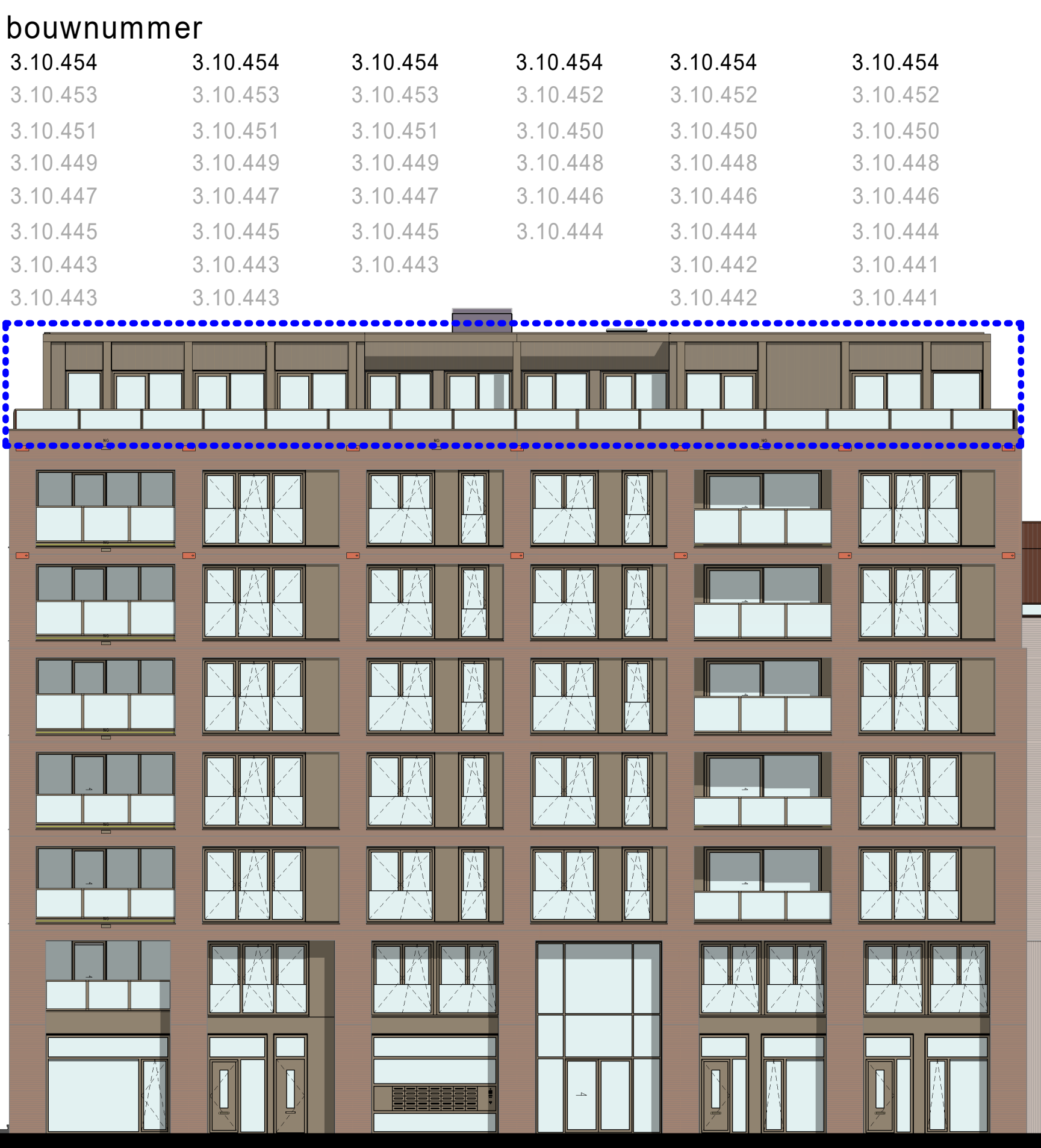
Noord-Oostgevel (Stratzijde) 1 : 150
