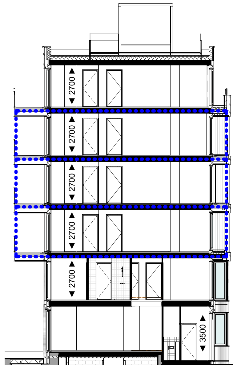
Doorsnede A-A
