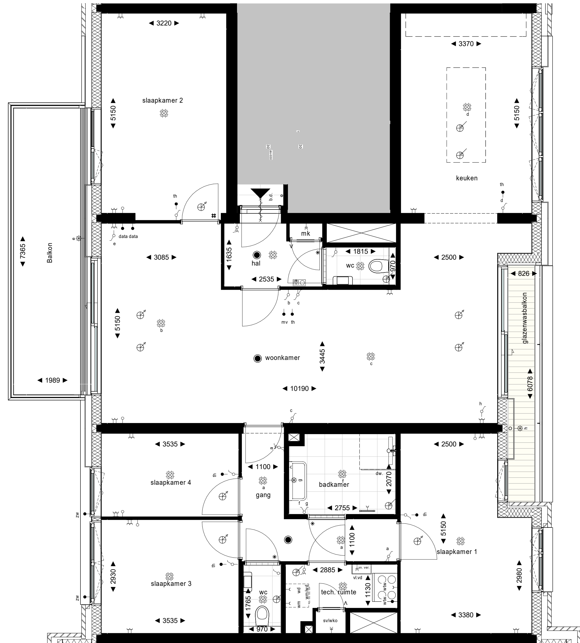
Tweede verdieping
