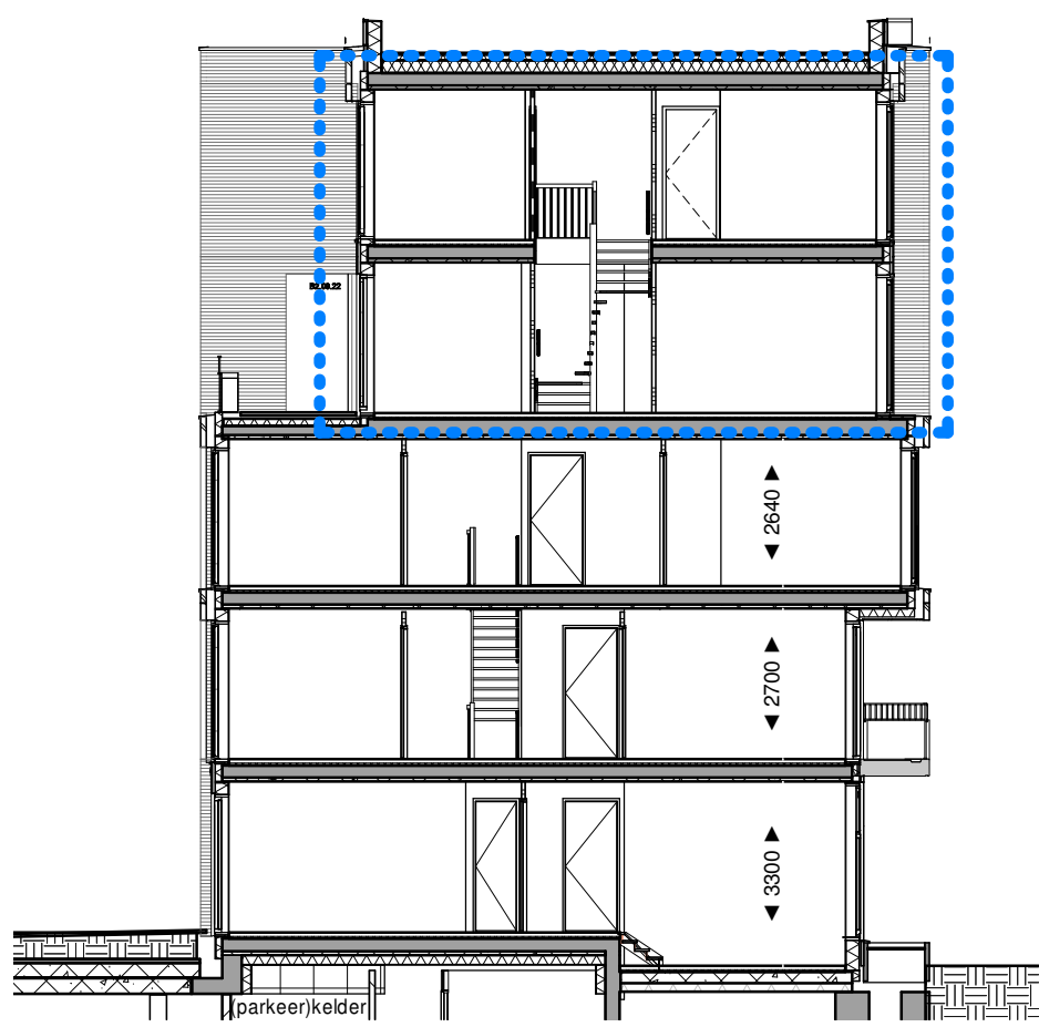
Doorsnede A-A 1 : 150
