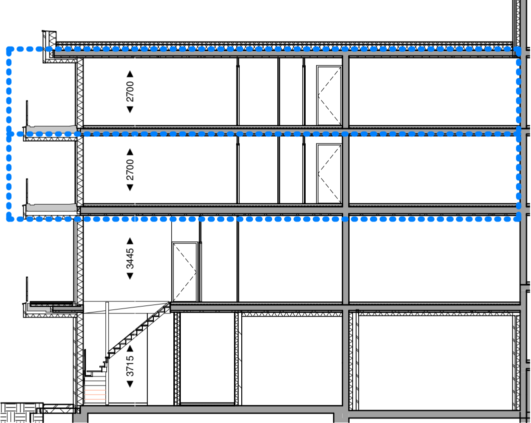
Doorsnede A-A
