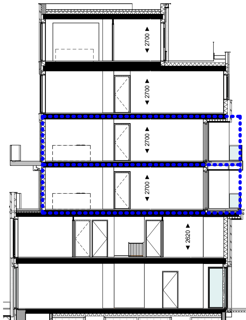
Doorsnede A-A 1 : 150
