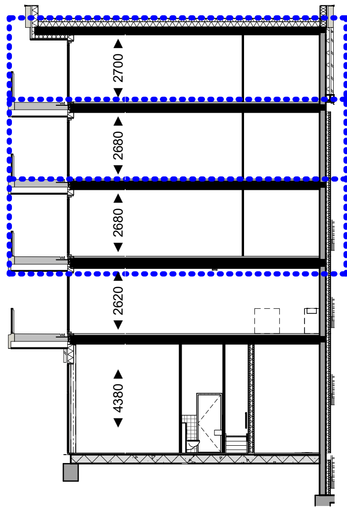
Doorsnede A-A
