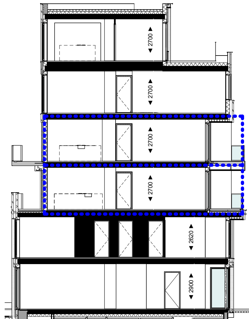
Doorsnede B-B
