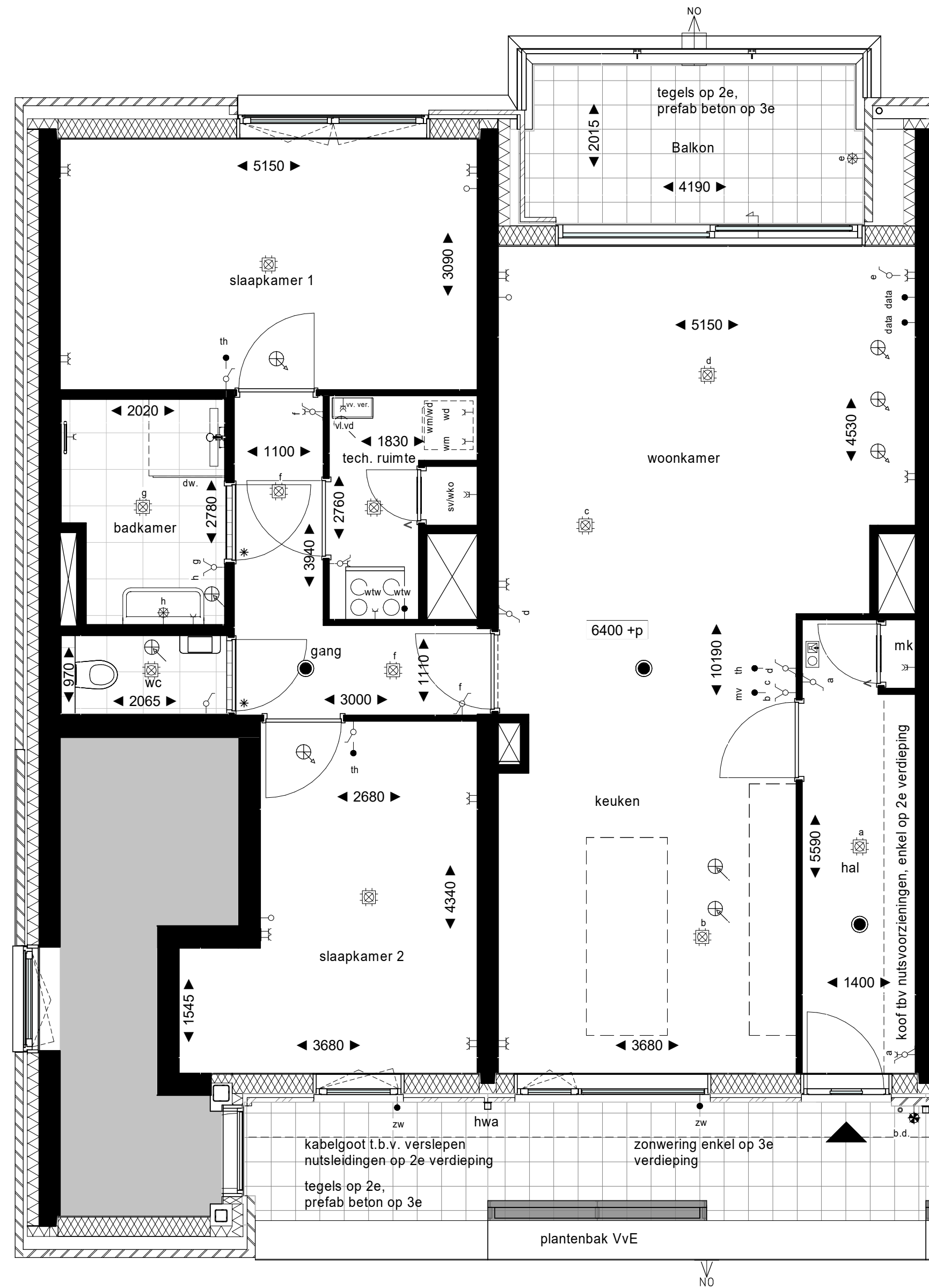
2e verdieping
