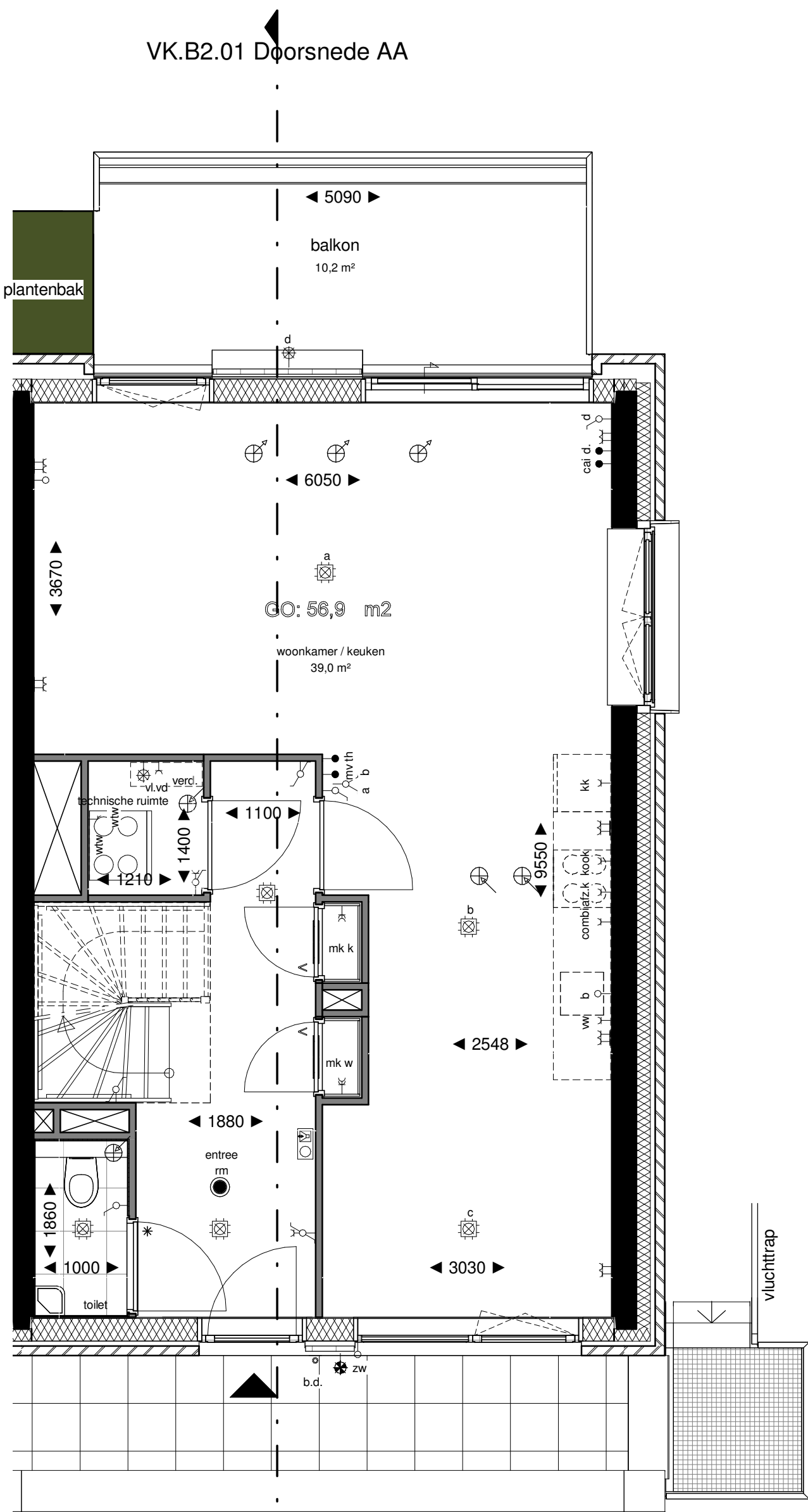
Derde Verdieping
