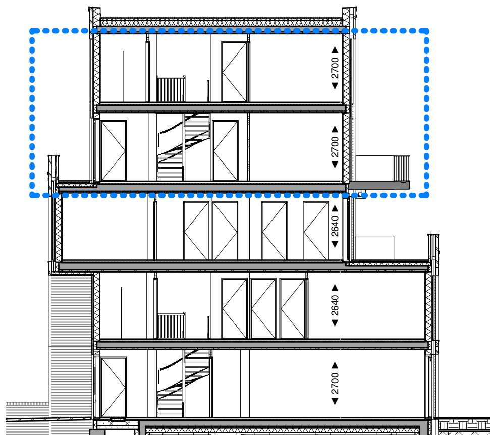
Doorsnede A-A
