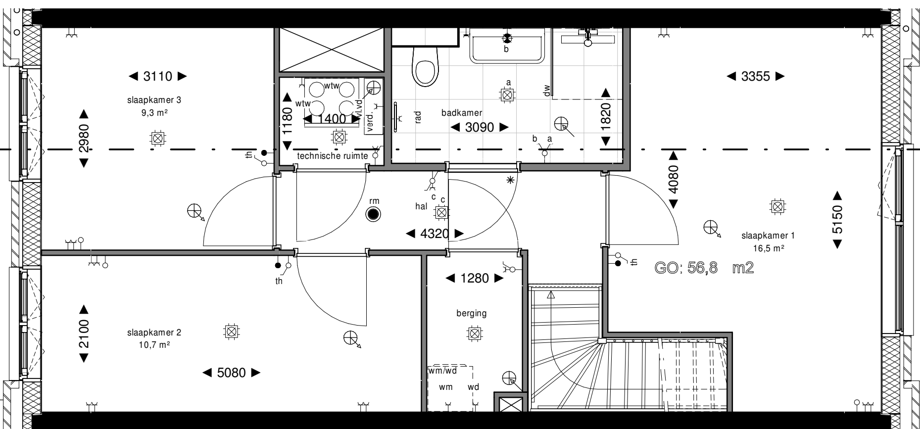
1e Verdieping
